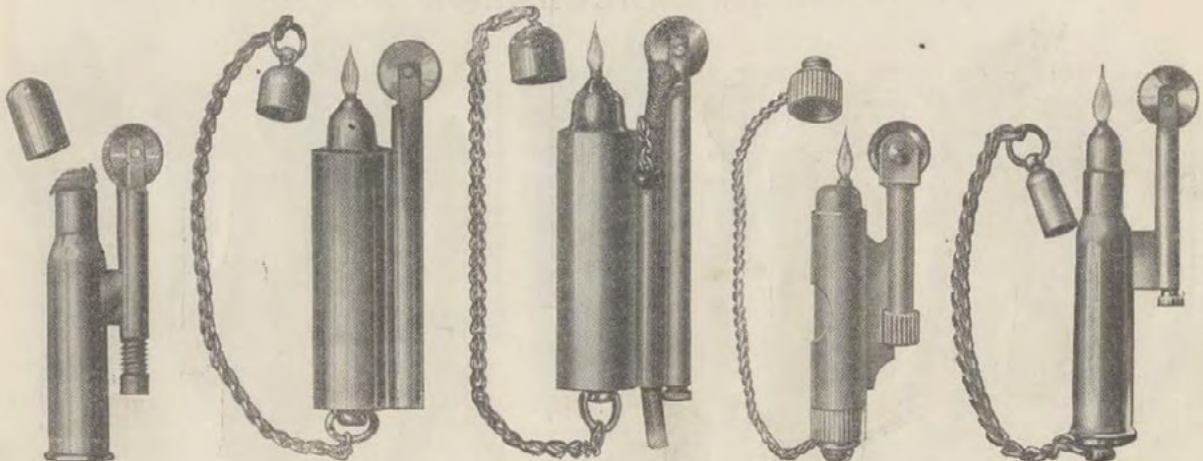
№ 51a. Огонекъ съ фитилемъ.
