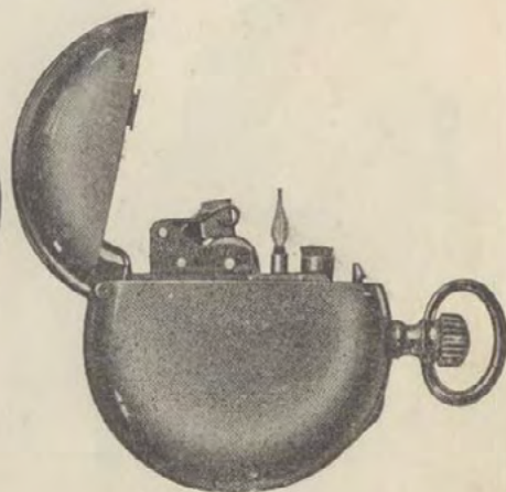
№ 83 "ЧЕМПИОНЪ". Дѣйствуетъ съ бензиномъ и безъ бензина. Весь легко разбирается. Весьма солидн. констр.
